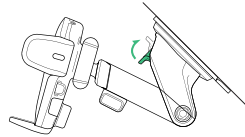
2. ロッキングレバーを押し下げ、吸着部に接着する。
